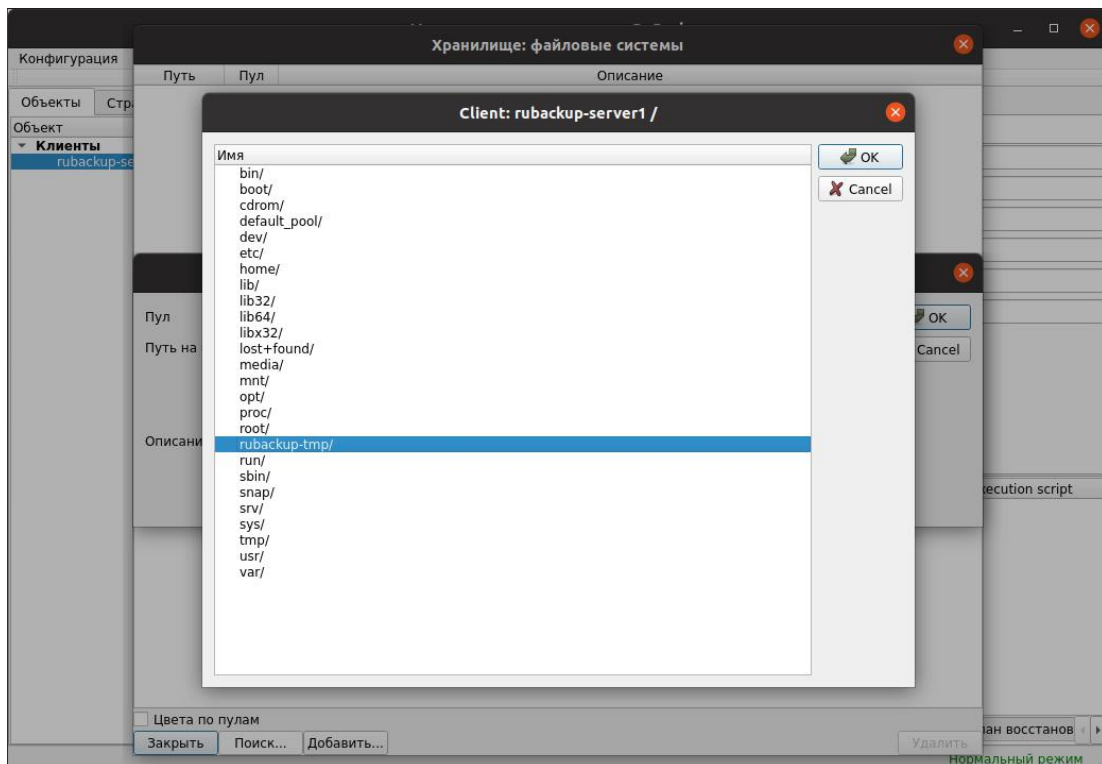
Рис. 3. Добавление локального каталога в качестве хранилища.
