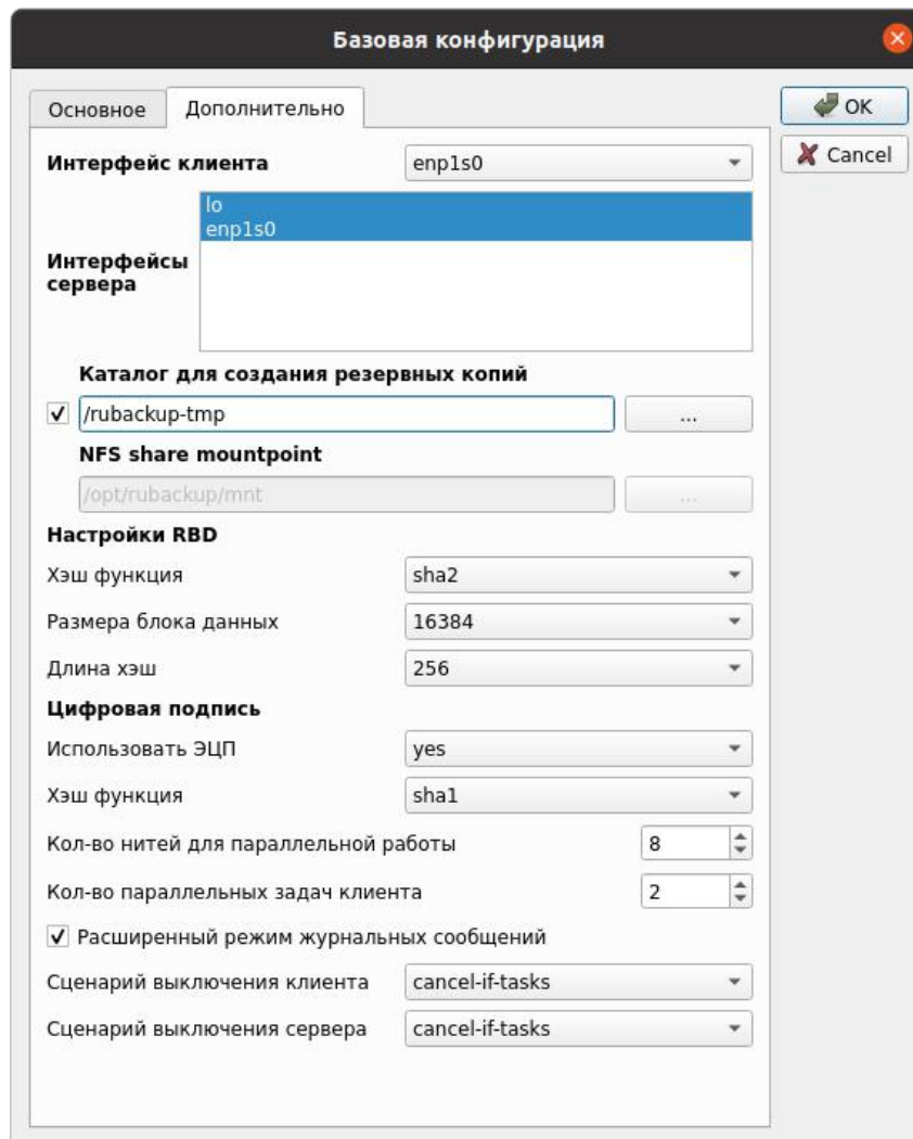
Рис. 5. Настройка временного локального каталога для хранения резервных копий.
